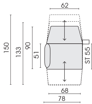
Funktionssessel breit drehbar AT links 172F
