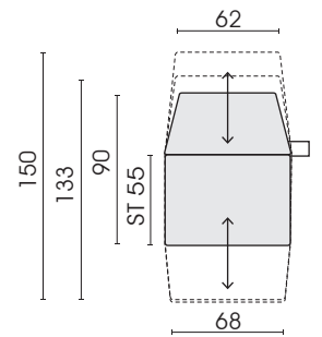
Funktionssessel breit drehbar ohne AT 173F
