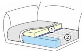
Taschenfederkern ① Schaum HR 38kg/m 3 ② Taschenfederkern
